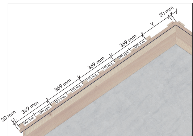
Vzdálenost latí u tašek Plano
