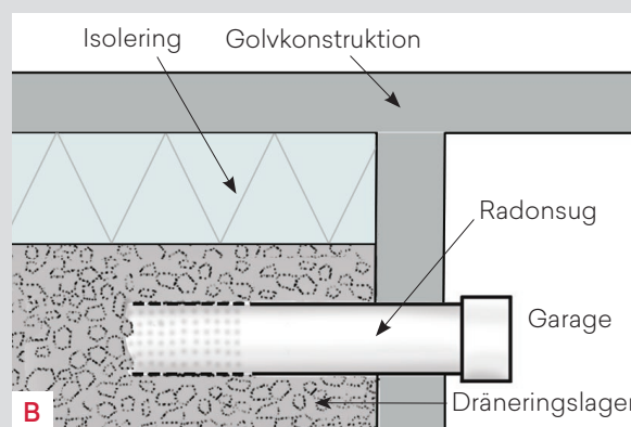
Princippskiss, horisontell montering under platta på mark
