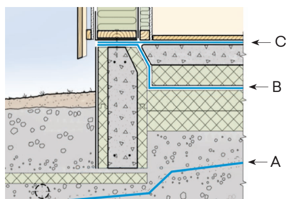
Alternativa placeringar (användargrupp) av radonspärr-/membran enl. SINTEF Byggeforsk.
