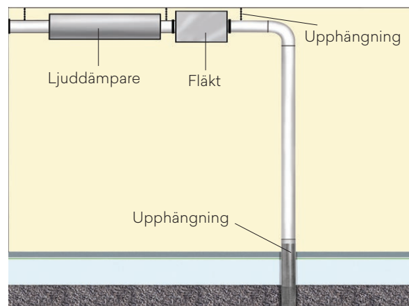
Principskiss, inkoppling av ventilation
