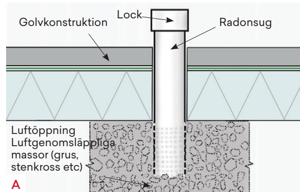
Principskiss, placering av radonsug
