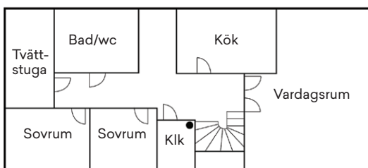
Exempel på placering av Radonsug i klädkammare
