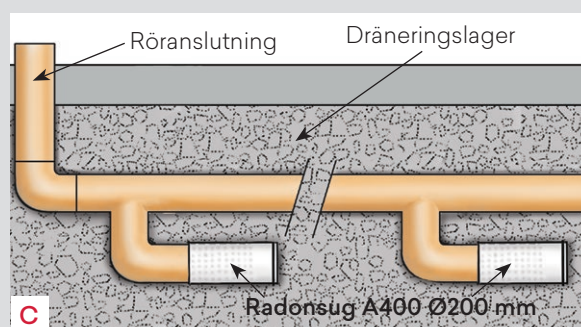
Princippskiss, montering av Radonsug A400 på större ytor
