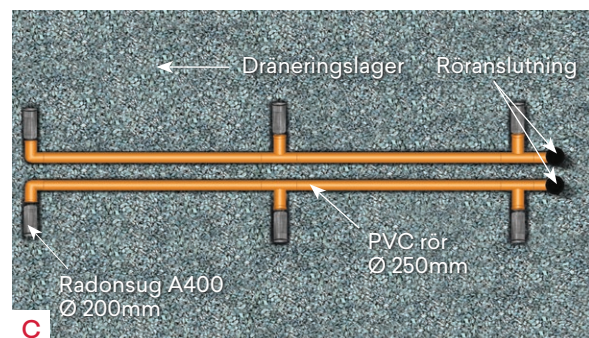
Principskiss, montering av Radonsug A400 på större ytor
