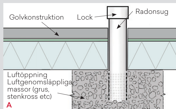
Princippskiss, placering av radonsug
