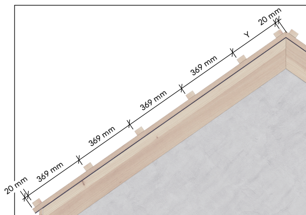
Traglattenabstände Nordic
