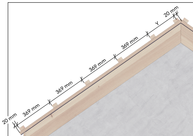
Traglattenabstände Plano
