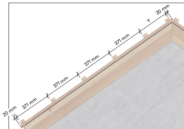
Traglattenabstände Exclusive
