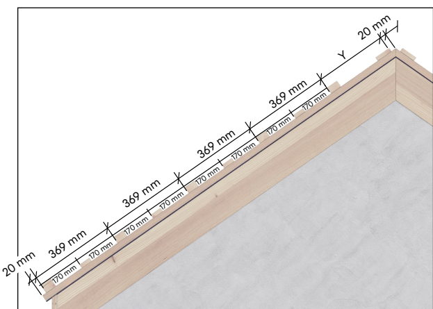
Traglattenabstände Plano
