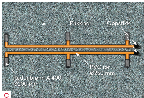
Prinsippkisse, montering Radonbrønn A 400 på større flater
