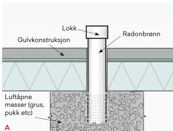
Prinsippkisse, plassering av brønn
