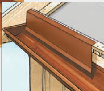
6.3.1 B Isola Takfotbeslag Powertekkplatene må festes i toppen (liten bølge) på nederste rad.
