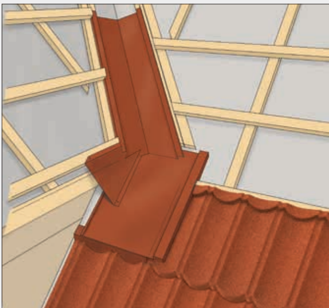
7.9.1C Kilrenneskuff 3
