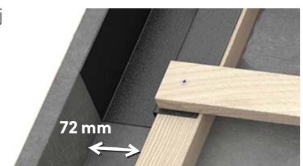
Skottrenne detalj
